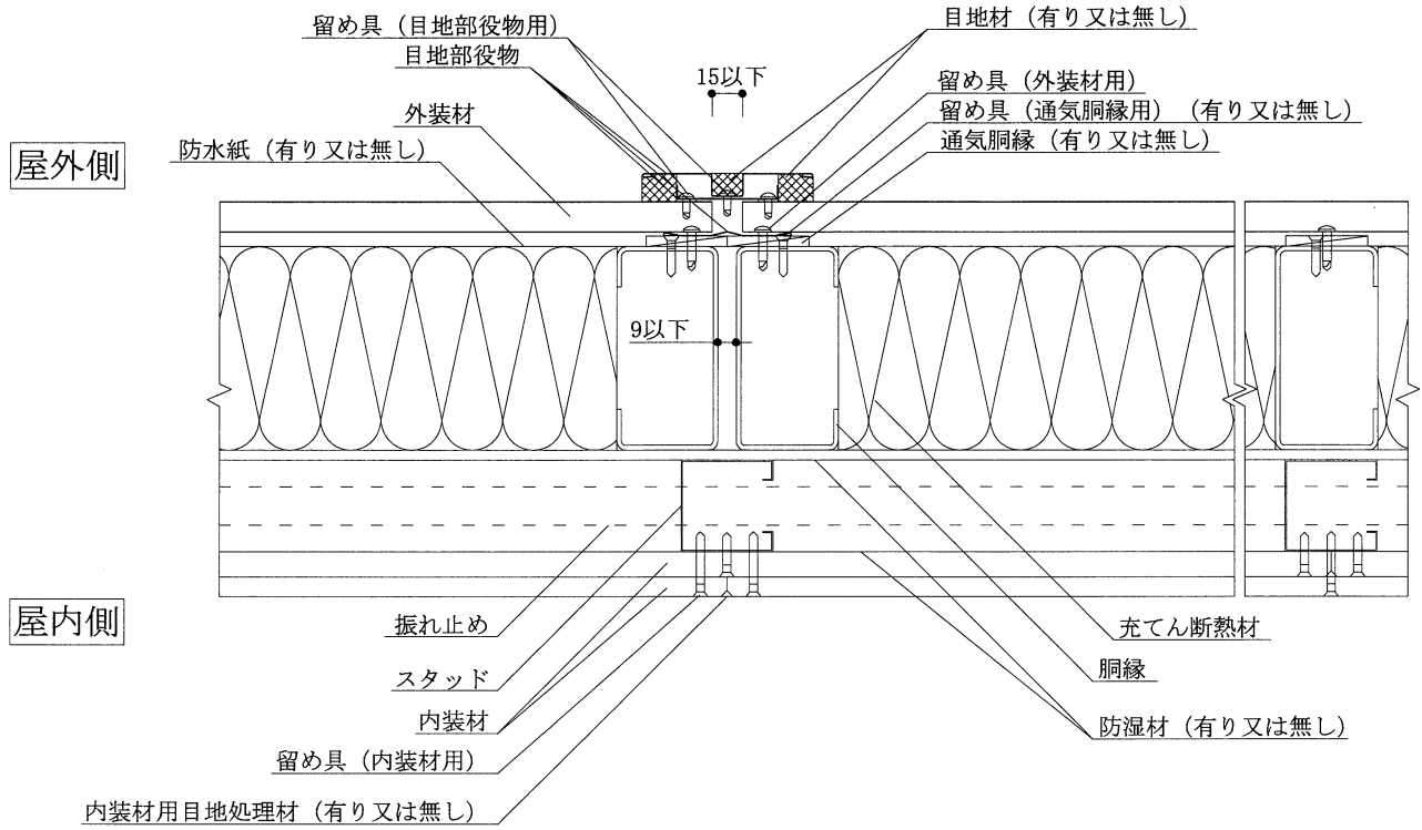
タイプ4 胴縁補助下地材無し
